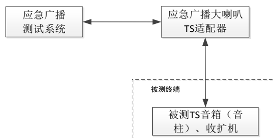
图F.30 TS 音箱（音柱）、收扩机测量框图
