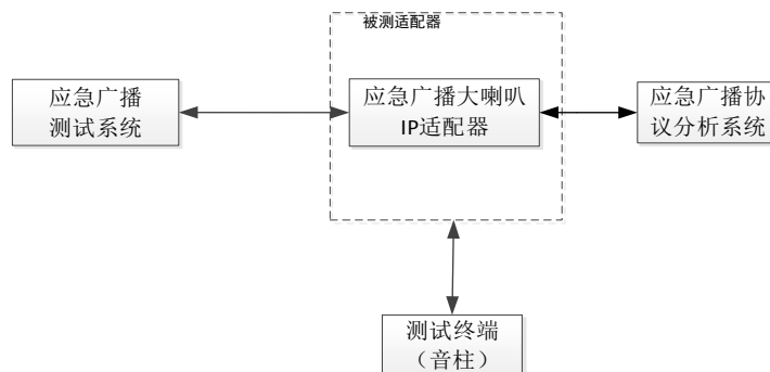
图F. 18 应急广播大喇叭 IP 适配器测量框图
